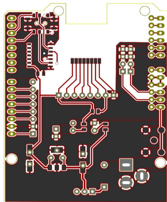
Figure 9 Top Guide Layer
